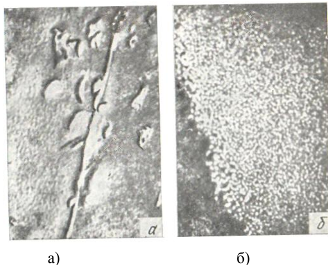
Рисунок 5 – Выделения фазы Al_3Li в сплаве 1420 после старения:
